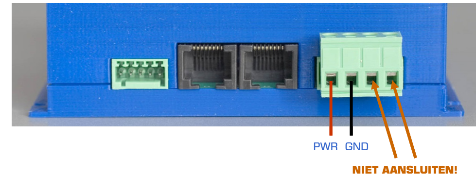
Fig 13: Aansluiten voeding op TM44
