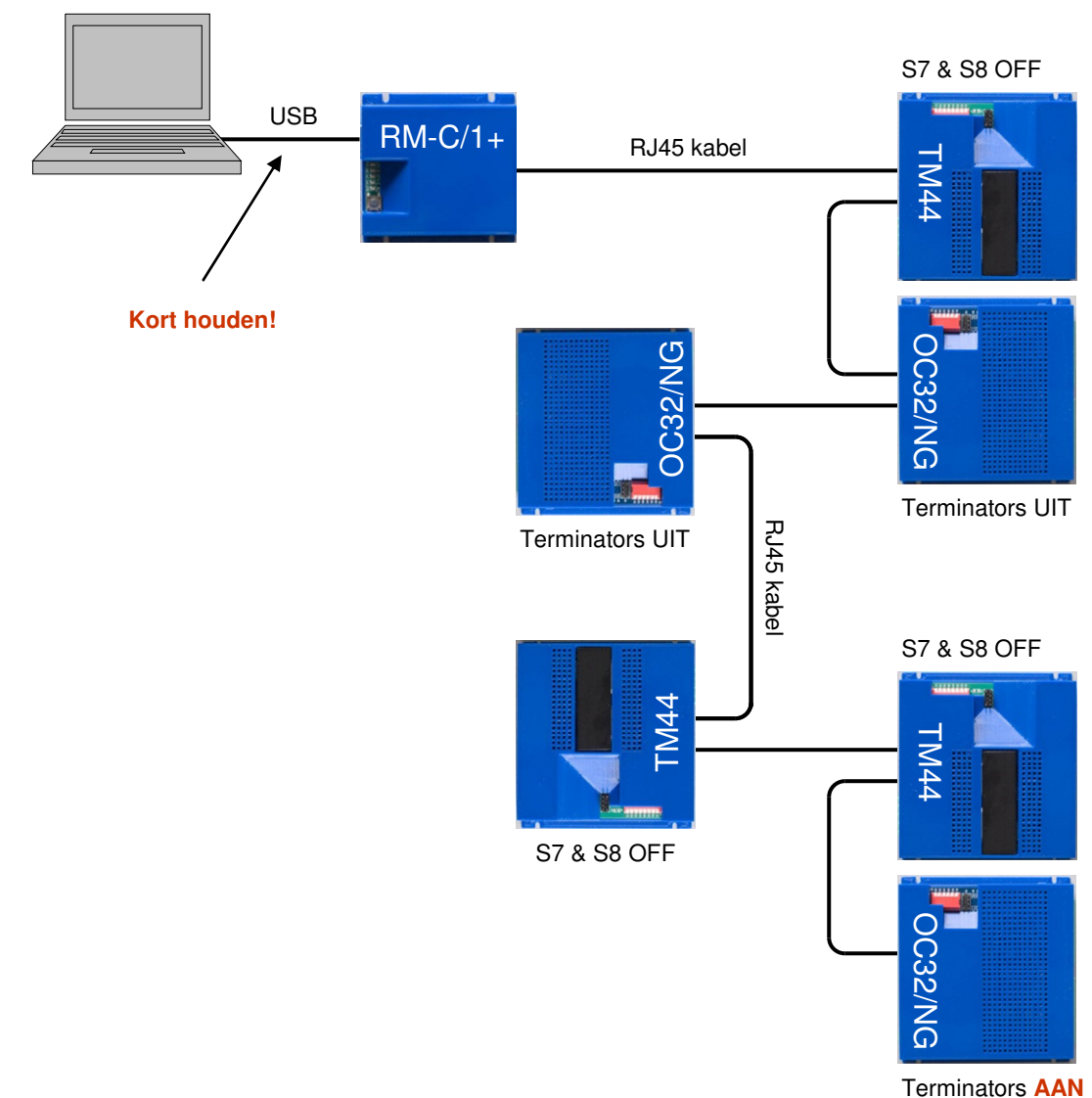
Fig 22: Nog een overzicht, nu met een OC32/NG als laatste module
