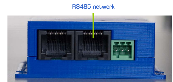
Fig 18: Netwerkaansluiting op RM-C/1+
