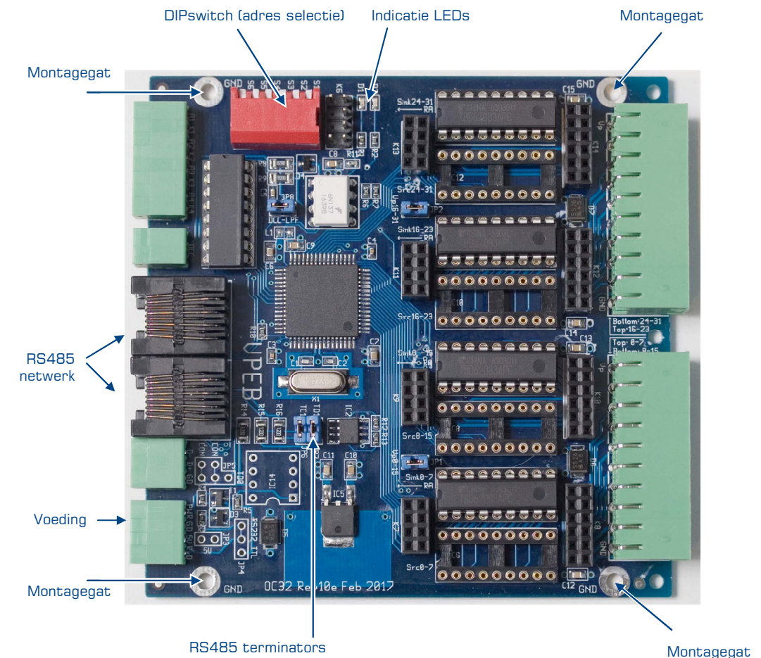
Fig. 16: OC32/NG overzicht
