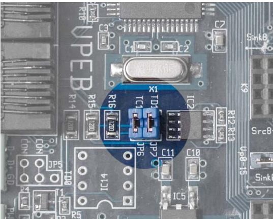
Fig 23: Terminator op de OC32/NG
