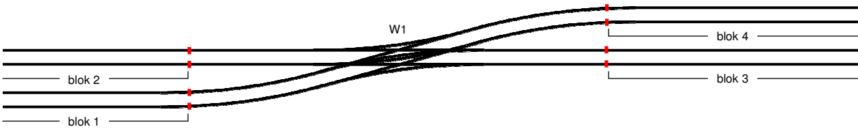
Fig 34: Engelse wissel
